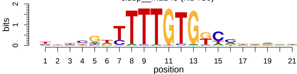
cisbp__M2148 (NDT80)
