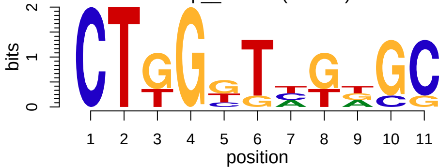
cisbp__M3079 (TFCP2)
