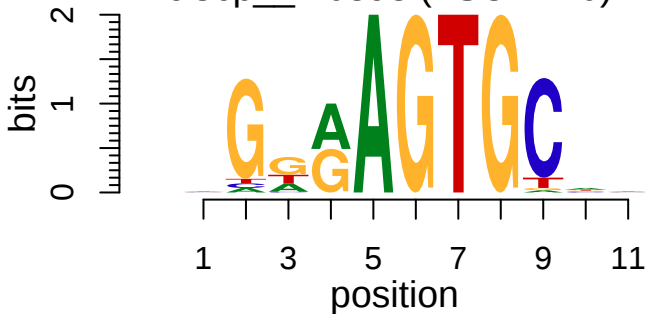
cisbp__M0398 (ZSCAN10)
