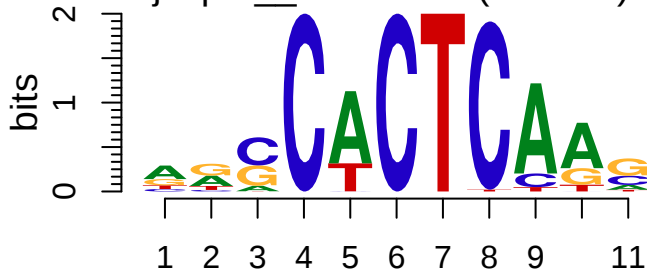
jaspar_MA0503.1 (Nkx2-5)
