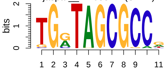
jaspar_MA0384.1 (SNT2)
