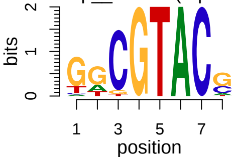
cisbp__M0438 (Zfp128)
