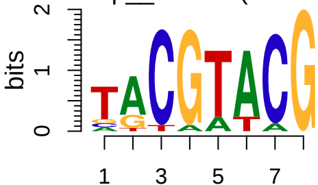
cisbp__M0606 (M0606)
