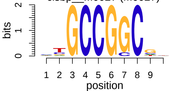
cisbp__M0027 (M0027)
