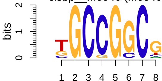
cisbp__M0040 (M0040)
