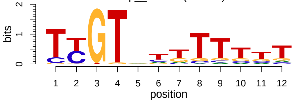
cisbp__M6251 (FUBP1)
