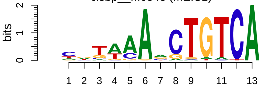
cisbp__M6343 (MEIS1)
