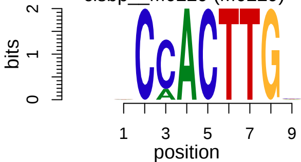
cisbp__M0229 (M0229)
