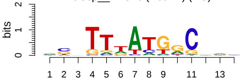
cisbp__M2526 (Abd-B) (RC)
